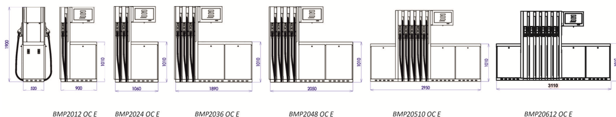
Рисунок 1. ТРК серии BMP 2000 ОС Е (EUROLINE)
