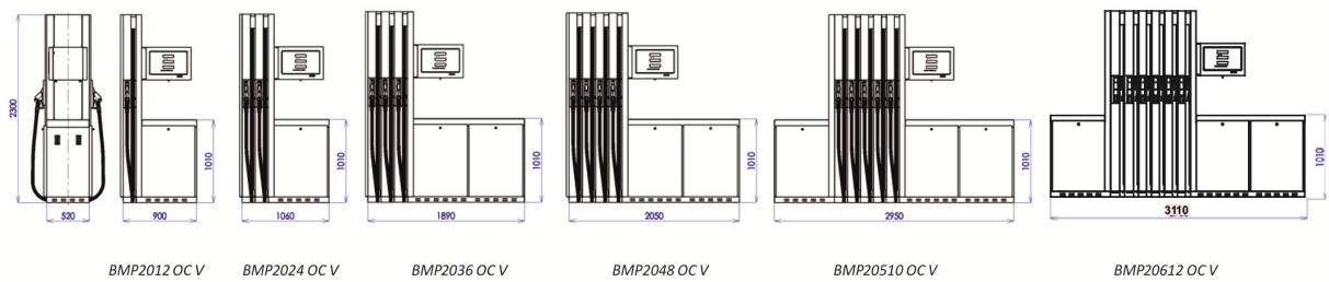
Рисунок 2. ТРК серии BMP 2000 OC V (VECTOR)
